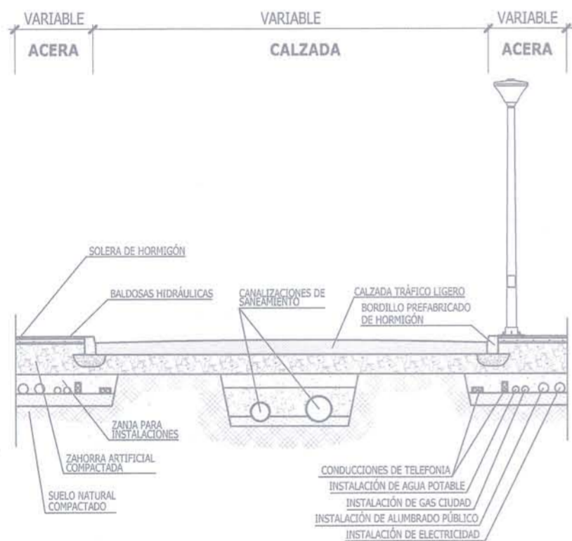
SECCIÓN TIPO CALLE S/E
