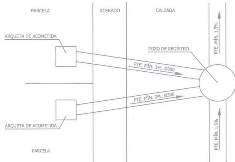
DETALLE DE ACOMETIDAS A PARCELAS S/E
