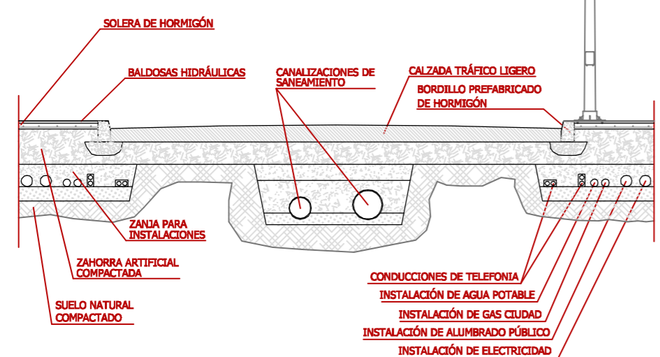
SECCIÓN TIPO CALLE S/E
