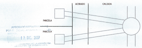
DETALLE DE ACOMETIDAS A PARCELAS E=1/50
