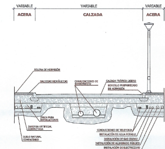
SECCIÓN TIPO CALLE SE
