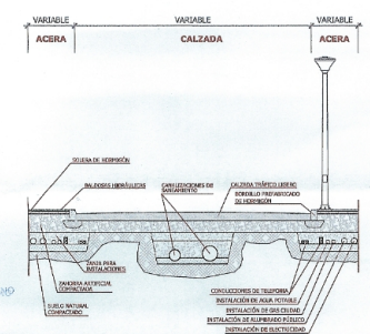
SECCION TIPO CALLE SE
