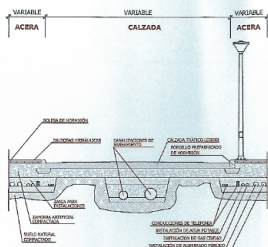
SECCIÓN TIPO CALLE - S/E
