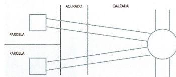
DETALLE DE ACOMETIDAS APARCELAS E=1/50
