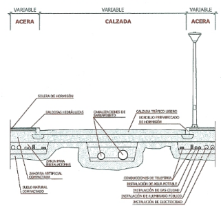
SECCIÓN TIPO CALLE 5/16
