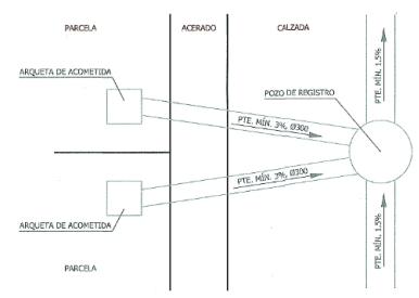
DETALLE DE ACOMETIDAS APARCELAS 6/156
