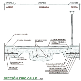
SECCIÓN TIPO CALLE SE
